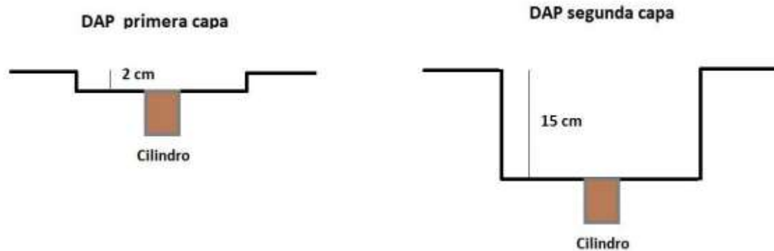
Figura 2. Muestreo de densidad aparente del suelo mediante el método del cilindro.
